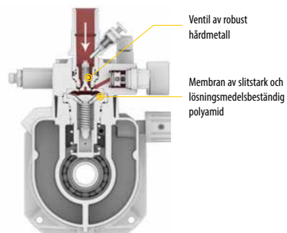
Fig: Membrandesignen ger en jämn och likformig rörelse av membranet. Det gör pumpen stabil och pålitlig.
